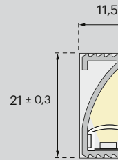
SECTION 1:1 (mm)
